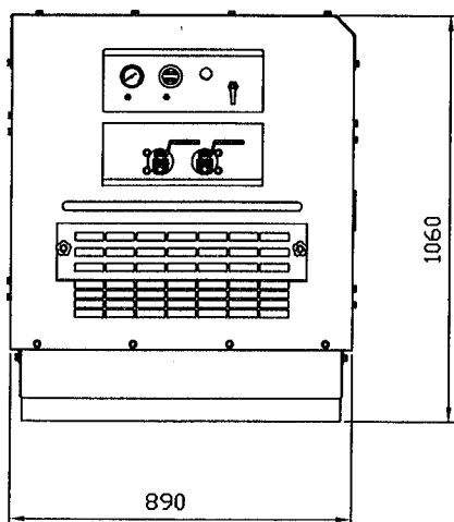
外形図
