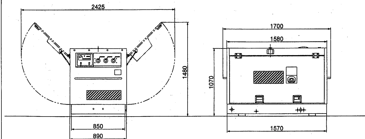
外形図
