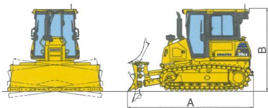
外形図
